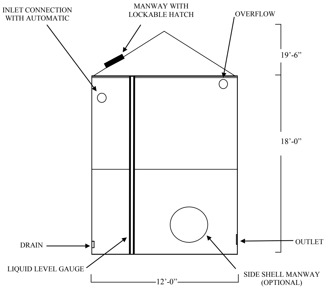
ELEVATION
